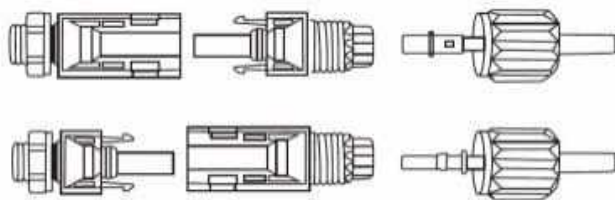
Рисунок 11 Сборка разъёмов PV
