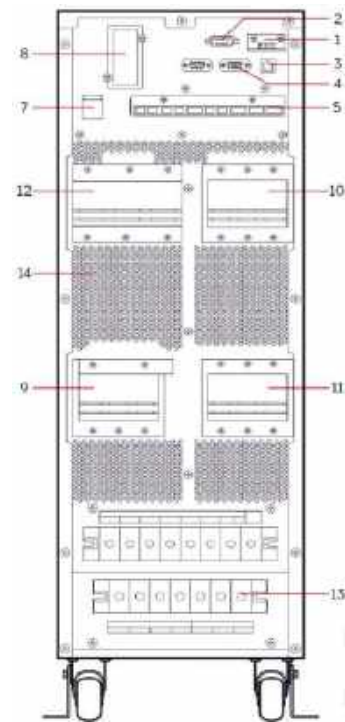
Рис. 1-7 Вид сзади 40 кВА
