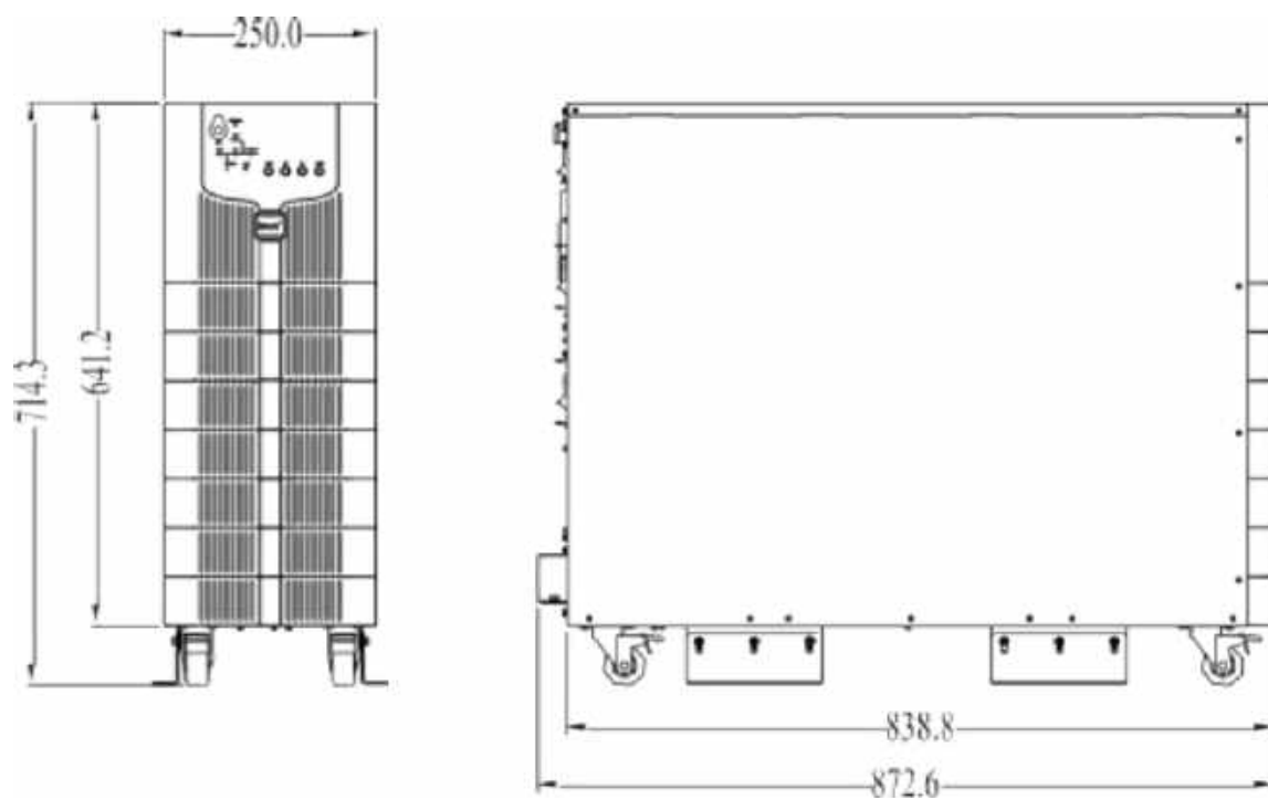
Рис. 11-1 Габаритные размеры ИБП
