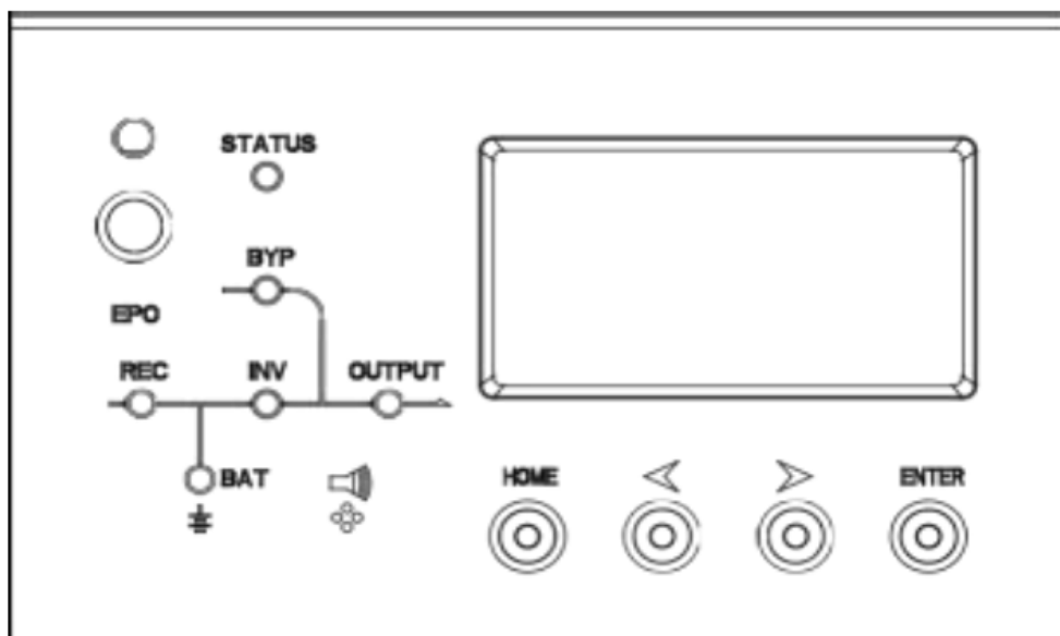
Рис. 5-1 Панель управления
