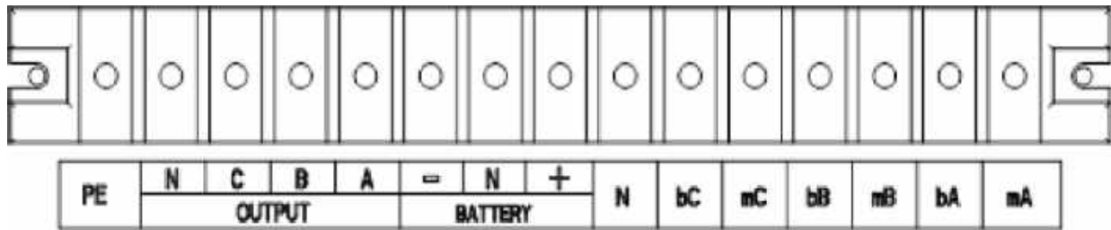
Рис. 4-1 Клеммная колодка 15кВА/20кВА
