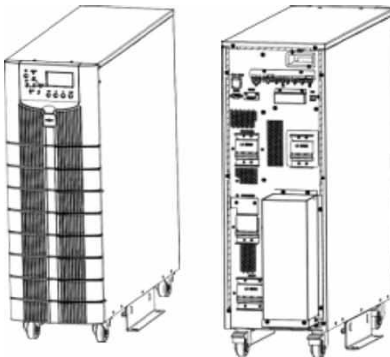
Рис. 1-1 Внешний вид
