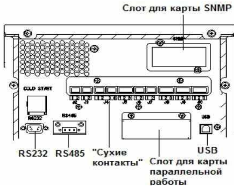
Рис. 4-2 Коммуникационные порты
