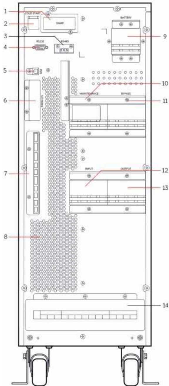
Рис. 1-2 Вид сзади
