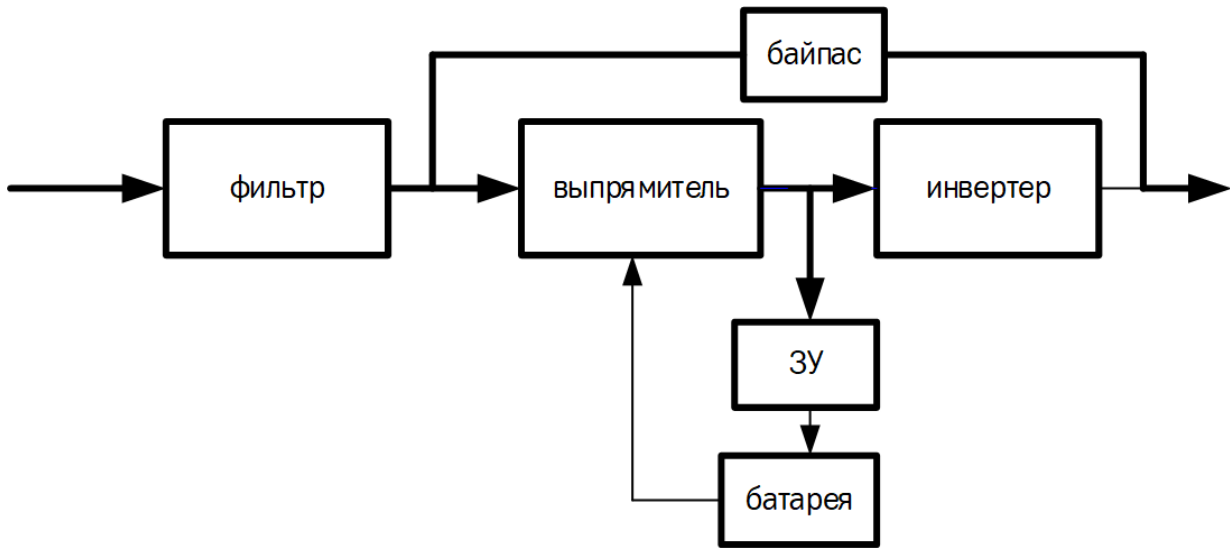
Рис. 3-5 ECO режим
