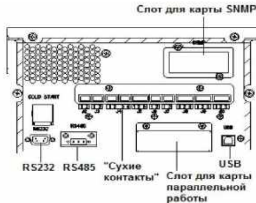
Рис. 4-4 Коммуникационные порты
