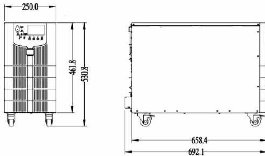
Рис. 11-1 Габаритные размеры ИБП 10/15 кВА
