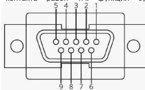
Рис. 7-1 DB9 порт
