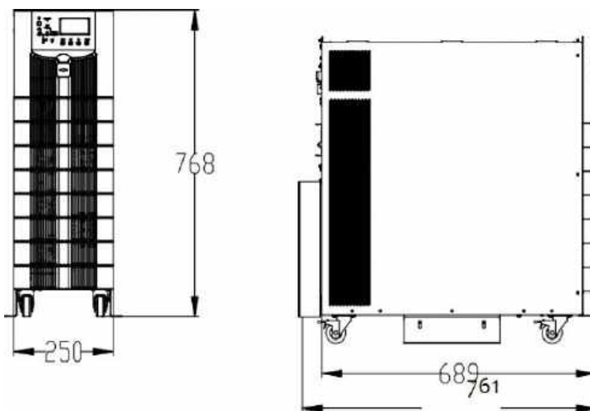
Рис. 11-3 Габаритные размеры ИБП 20/30 кВА
