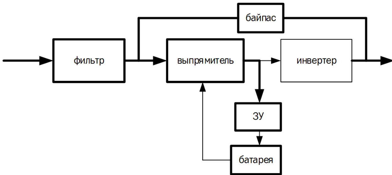
Рис. 3-3 Режим байпаса
