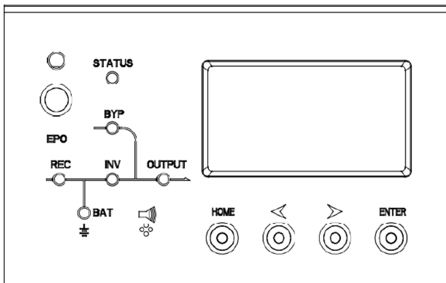
Рис. 5-1 Панель управления
